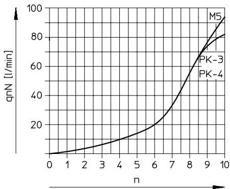
Caudal nominal normal q_{nN} con 6 → 5 bar en función de las revoluciones del husillo n
