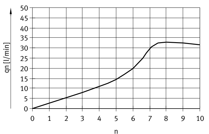
Caudal normal q_n con 6 → 0 bar en función de las revoluciones del husillo n
