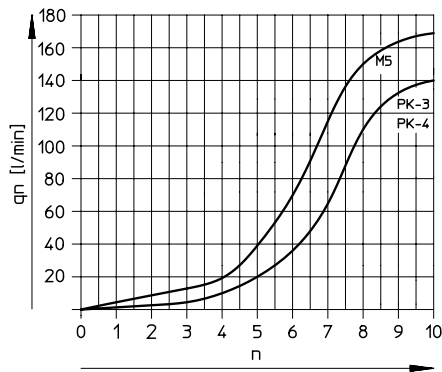
Caudal normal q_n con 6 → 0 bar en función de las revoluciones del husillo n
